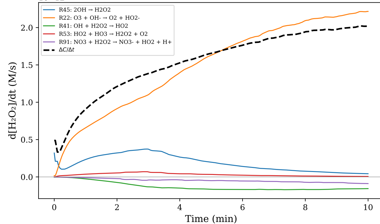
(d) \text{H}_2\text{O}_2
